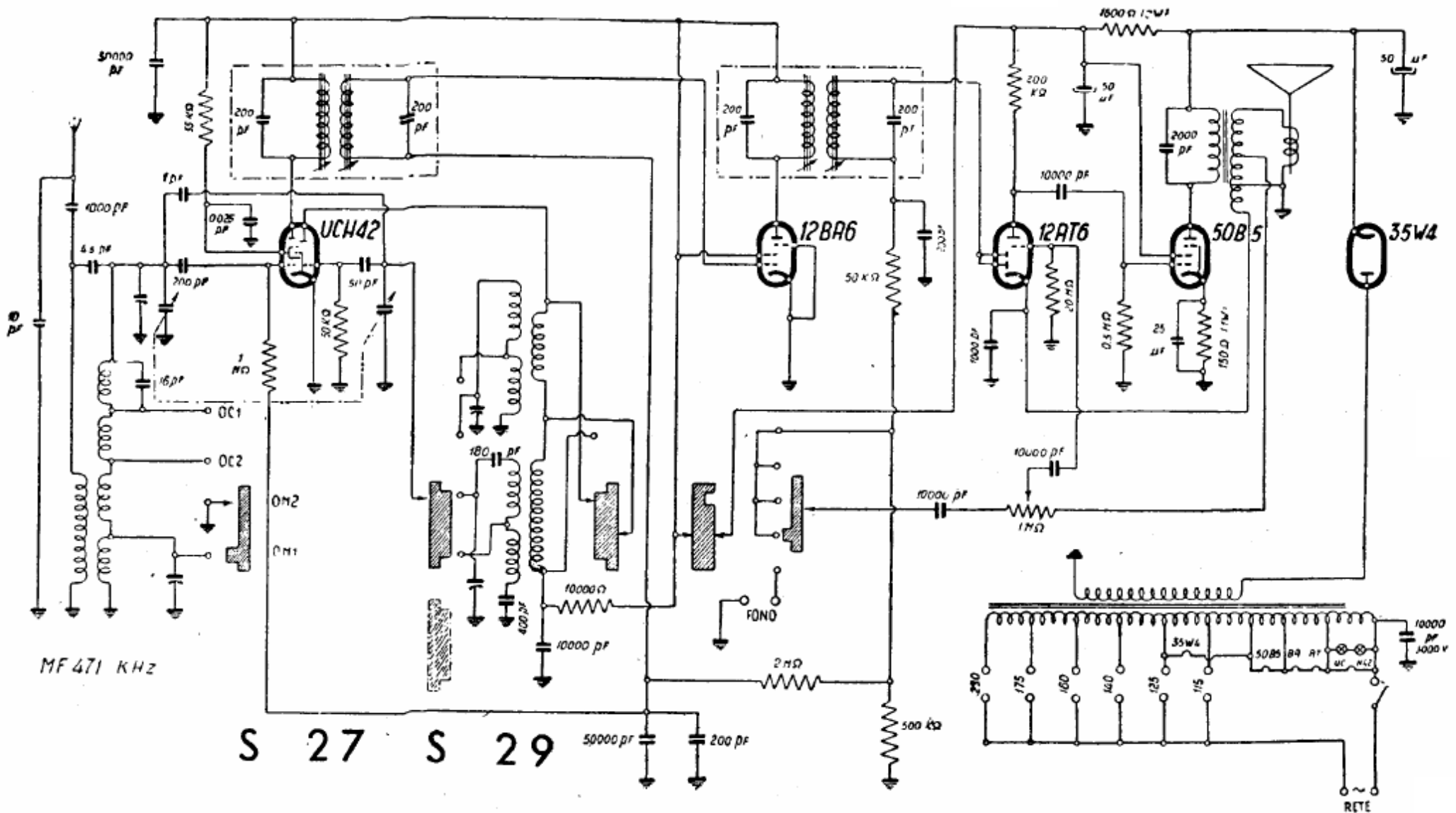
MAGNADYNE RADIO - Modd. S 27 e S 29 - Onde medie divise e due gamme onde corte. Media frequenza 471 kc. Reazione inversa dal secondario del trasformatore d'uscita. Potenza d'uscita 2 watt.
